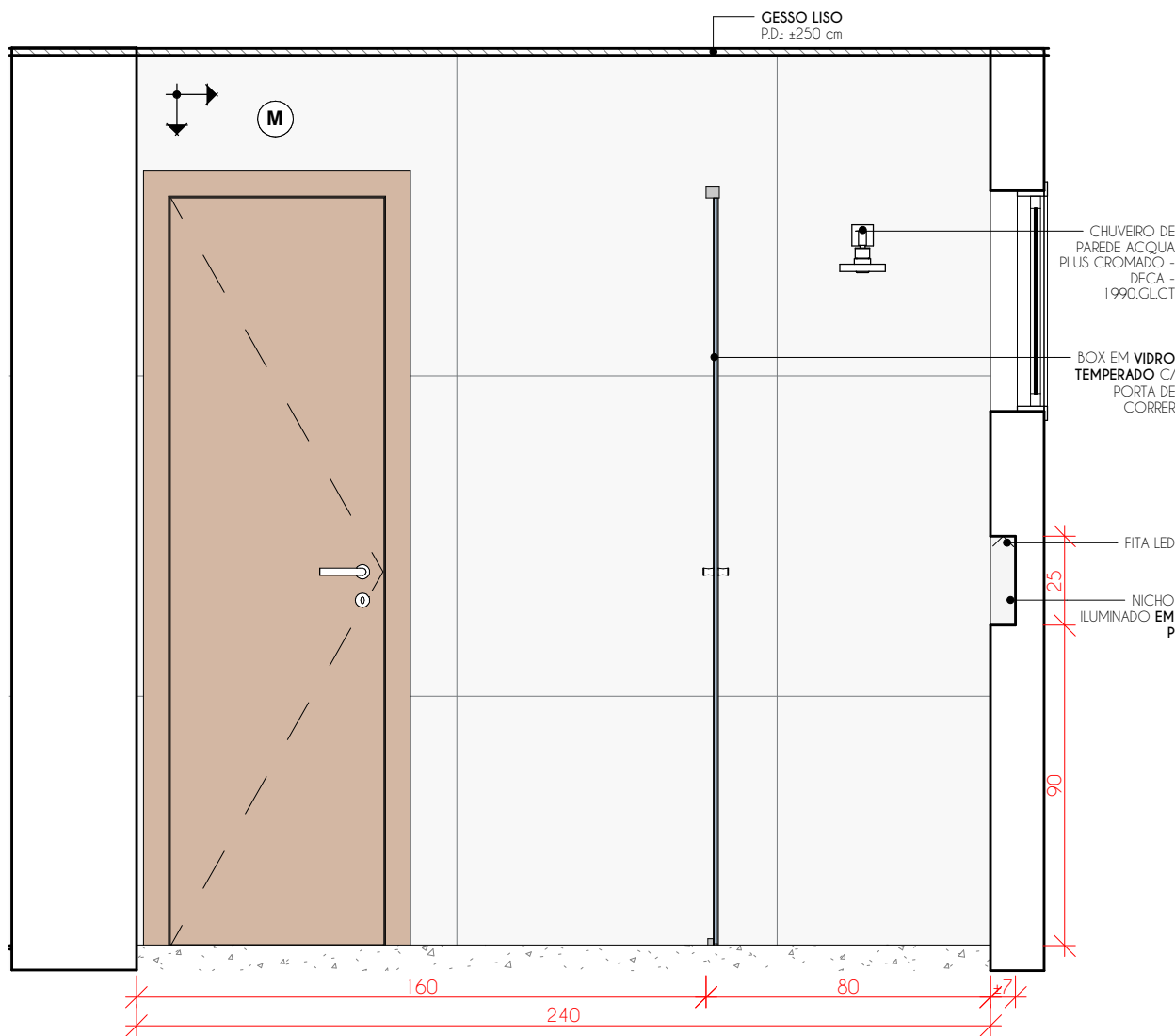
VISTA C ESCALA 1 : 20
