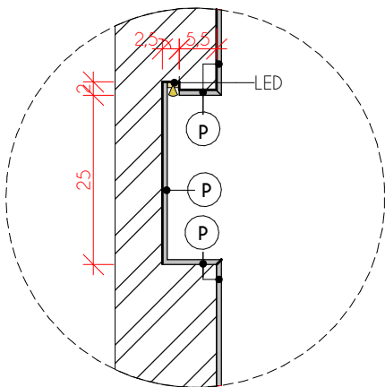
CORTE BB ESCALA 1 : 10
