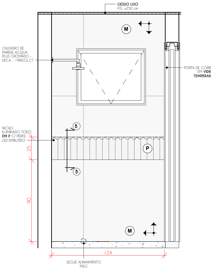
VISTA D ESCALA 1 : 20
